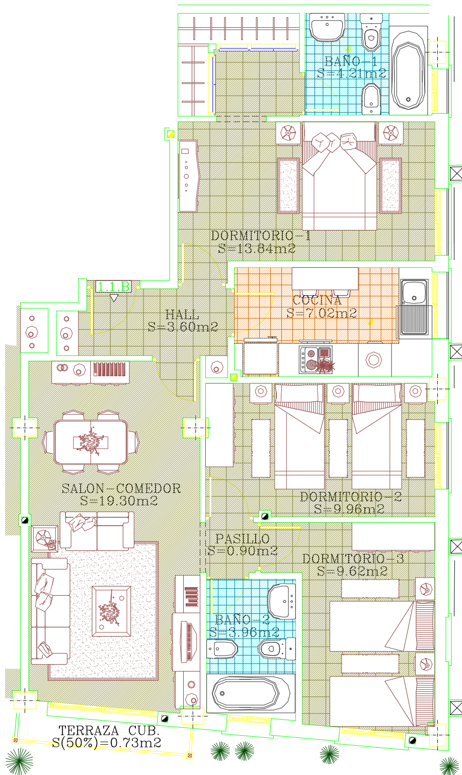
PISO 1.1.B. DE 3 DORMITORIOS
